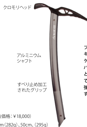
クロモリヘッド
